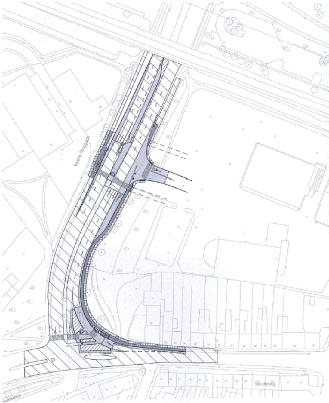
Tegning som viser signalreguleret T-kryds og shunt fra Tøndervej til Vestre Ringgade.
