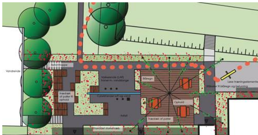
Detailudsnit af arealet ved hjemmeplejens bygning viser en cykellounge og opholdsplads.
